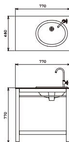
ガーデンシンク スタイル L シルバー 人工大理石 (ガーデンボウル無地)
