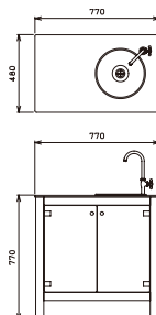
ガーデンシンク エレガント L シルバー 人工大理石 両扉 (ステンレスボウルS)
