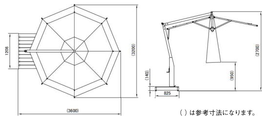
■ 基本寸法図 (mm)
