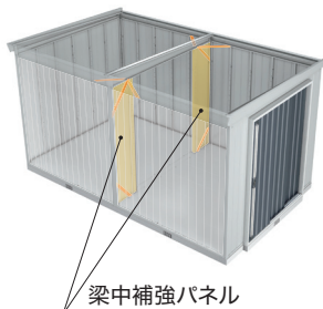
梁中補強パネル
