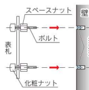
タップボルト M3×40L ×2本
