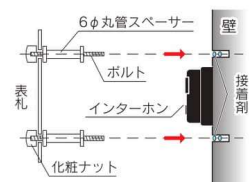
インターホンサイン・インターホンカバー用 化粧ボルトセット (M4 ボルト)
