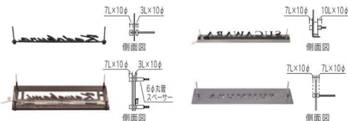
化粧ボルト M4×60L ×2~4本
